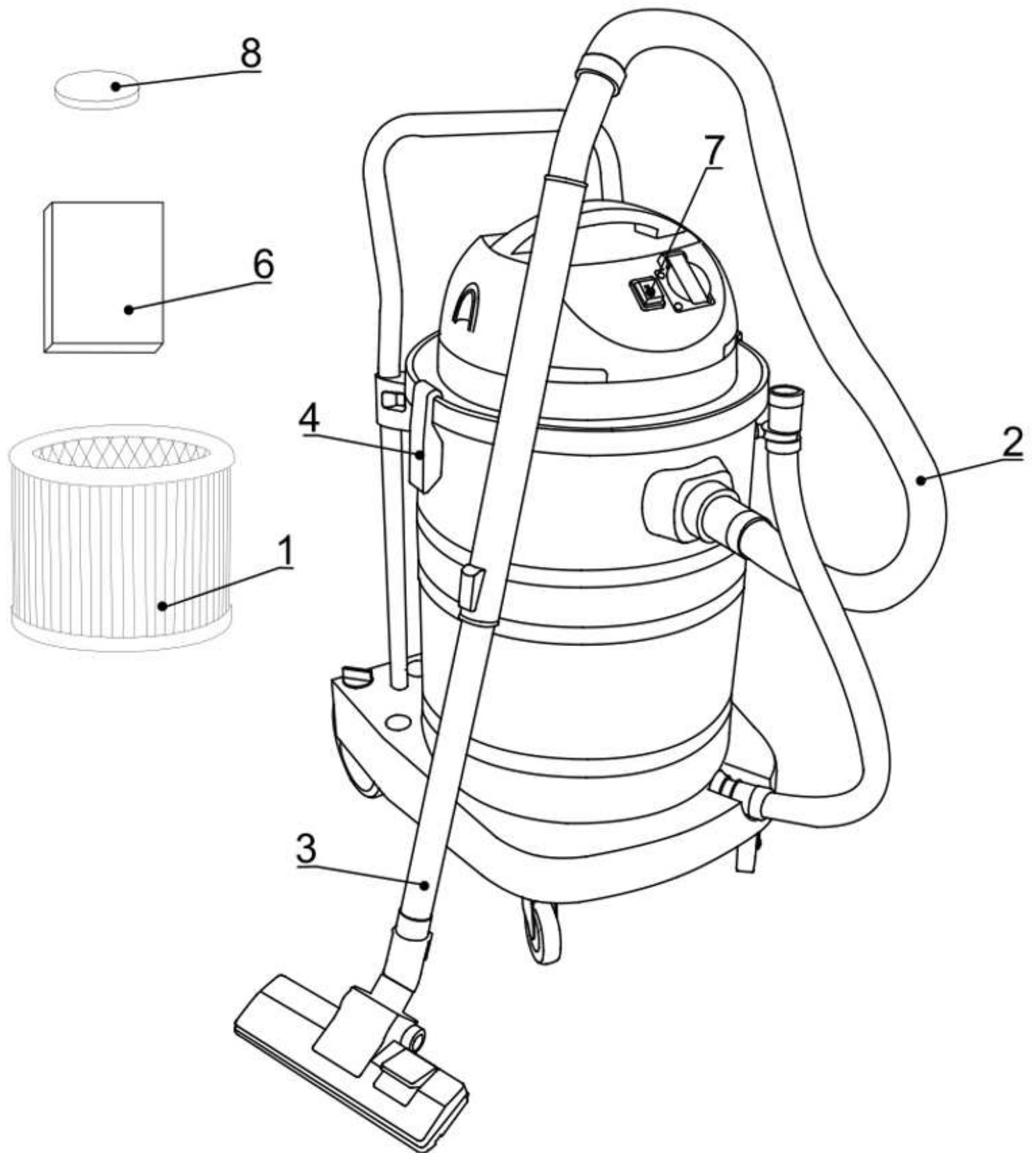
Odkurzacz POW0348 Rysunek 1/1
