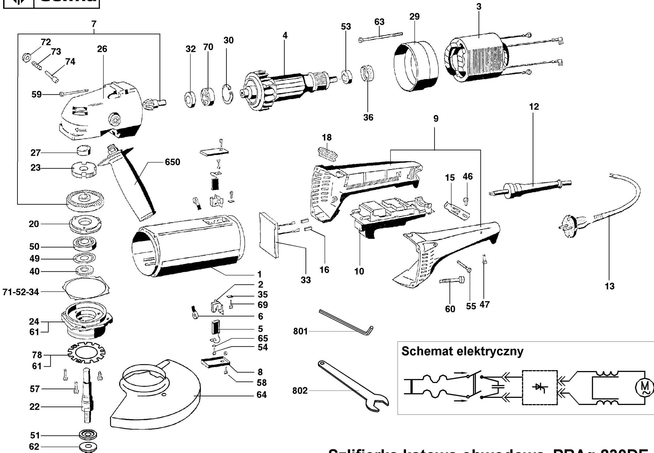
Szlifierka kąтова obwodowa PRAg 230DE
