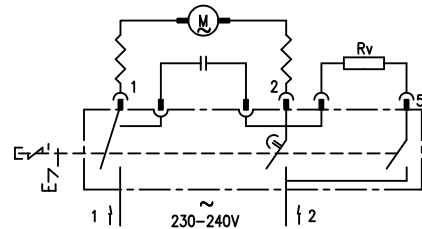
Schemat elektryczny 230÷240 V
