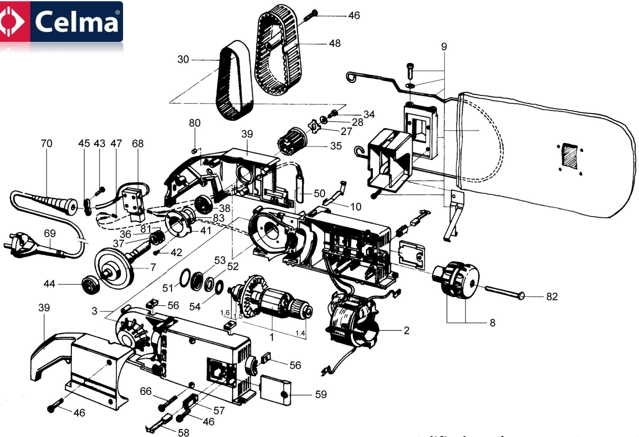
Szlifierka taśmowa DBSMm 75C
