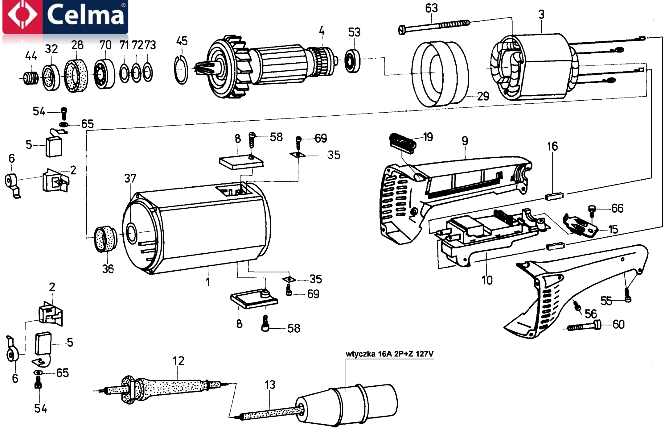
Szlifierka kątowna do pracy na mokro PRAW 130A
