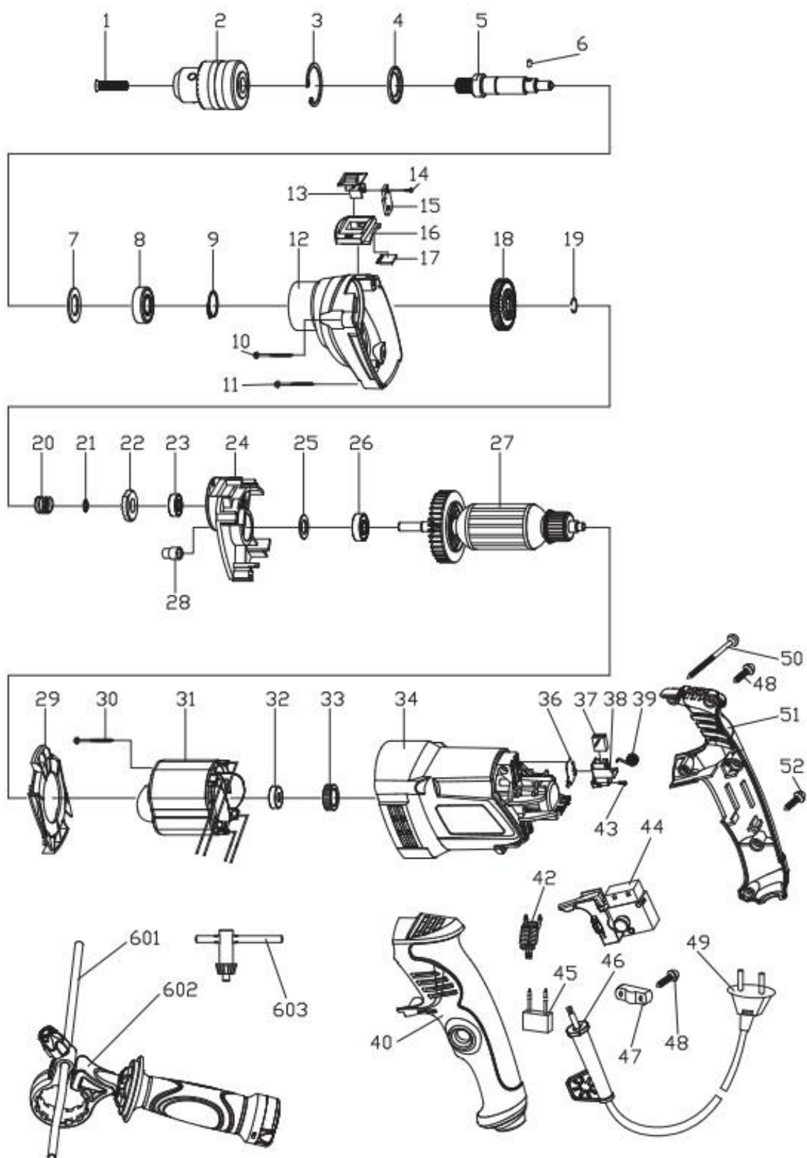
Wiertarka udarowa PRCm 13 GEO
