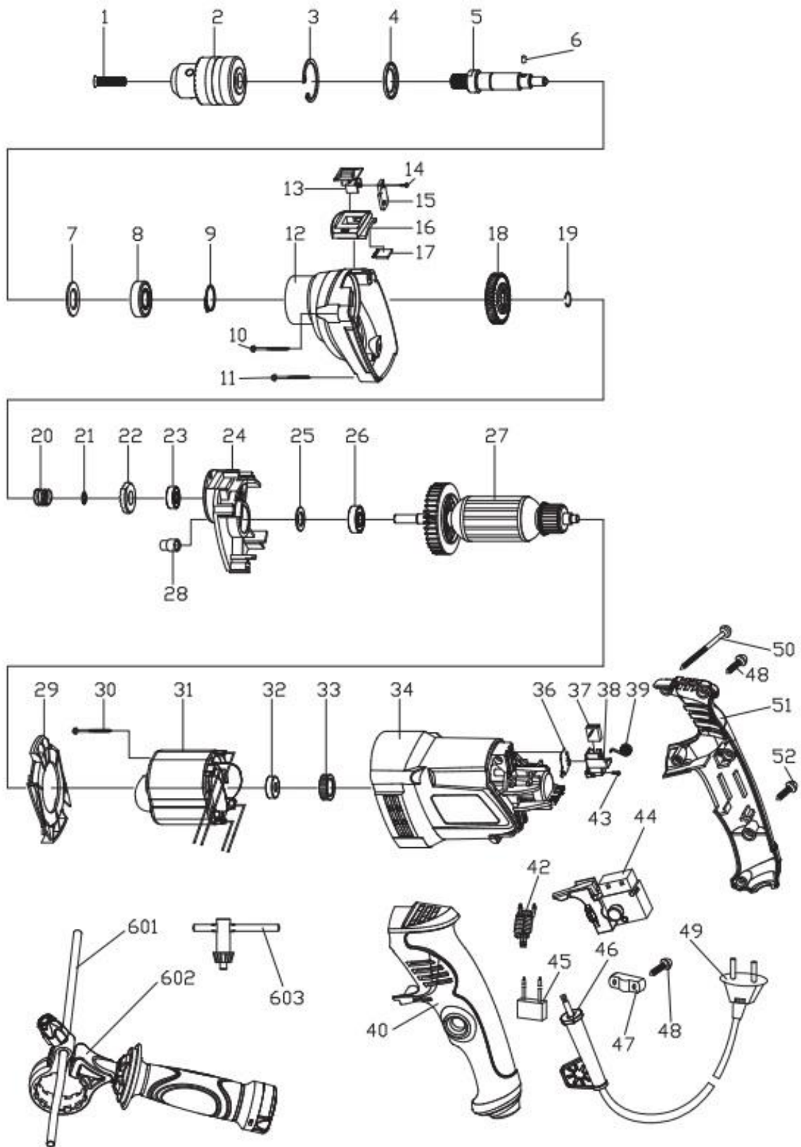
Wiertarka udarowa PRCm 13 IEO
