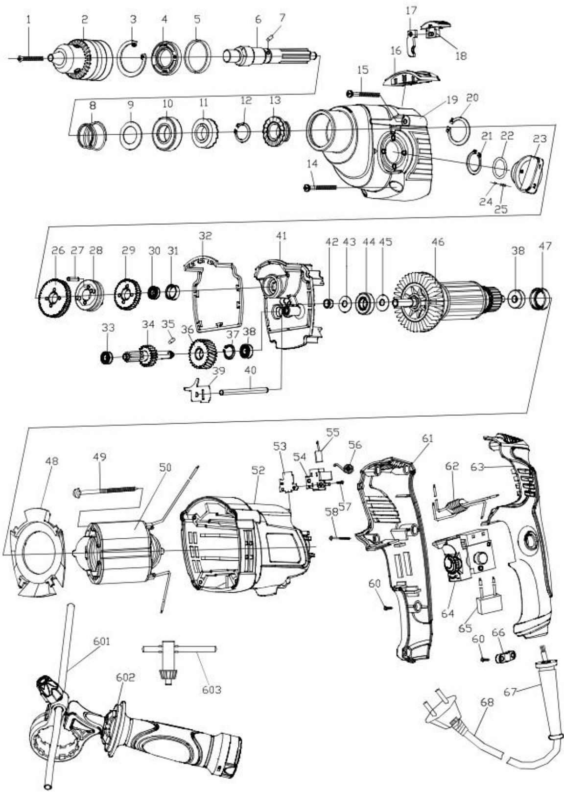
Wiertarka PRCz 13 GEO
