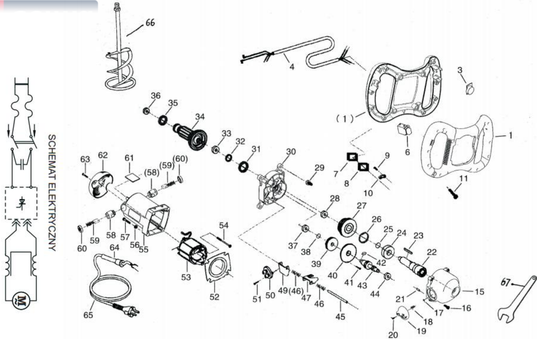
Mieszarka PRDa 140 AEO
