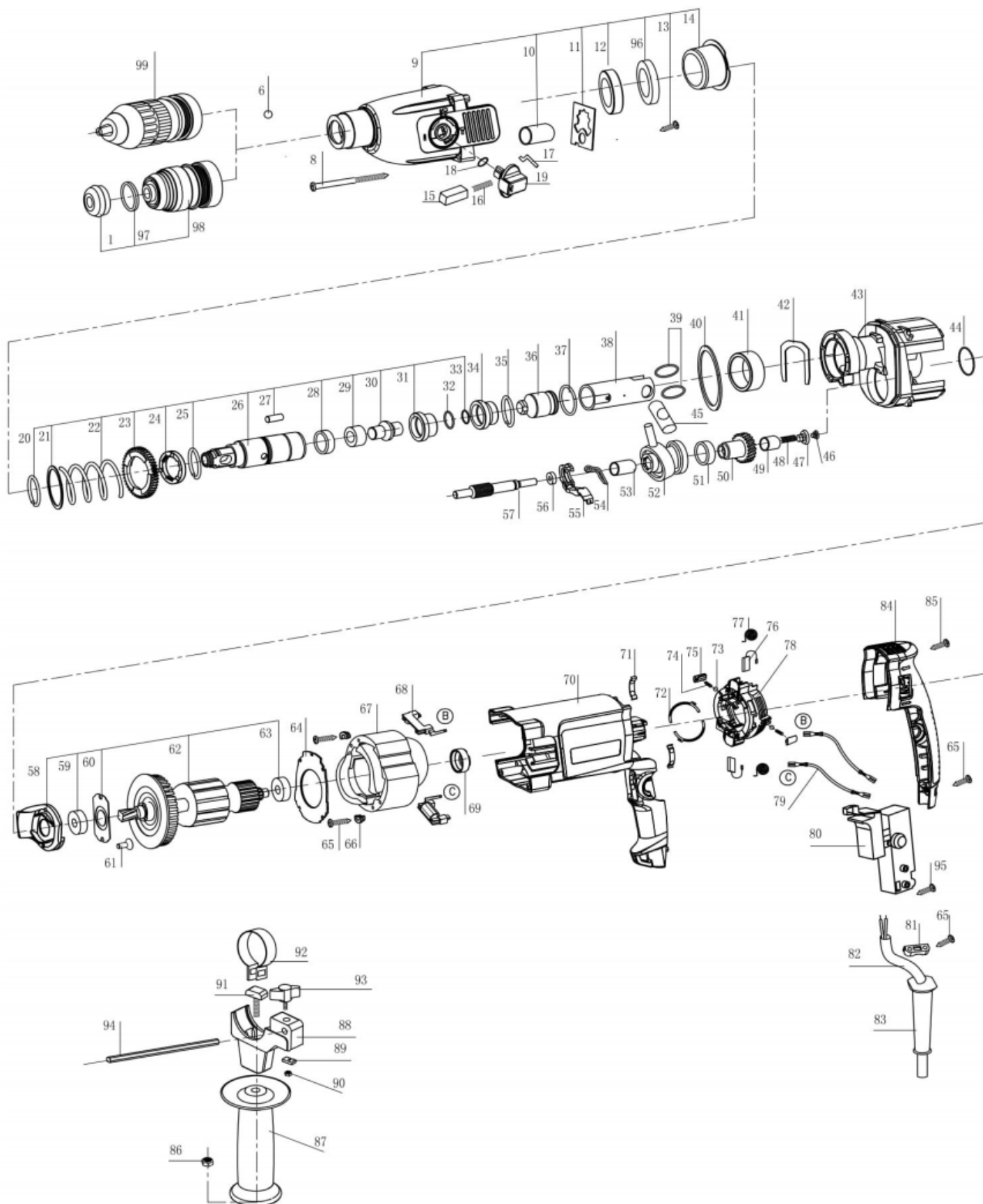
Młot udarowo-obrotowy PRWg 30 IEO
