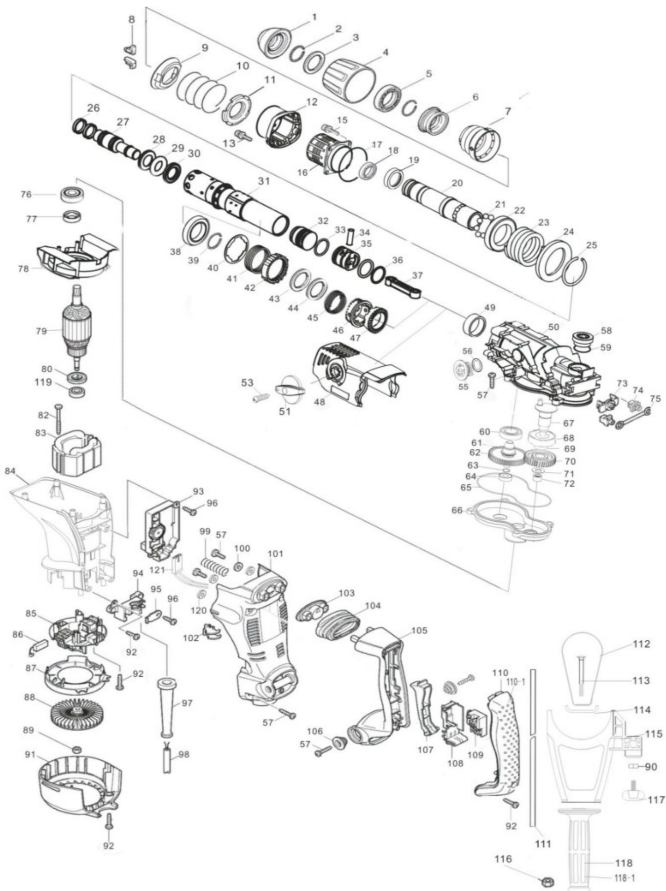
Młot udarowo-obrotowy PRWg 40 IEO
