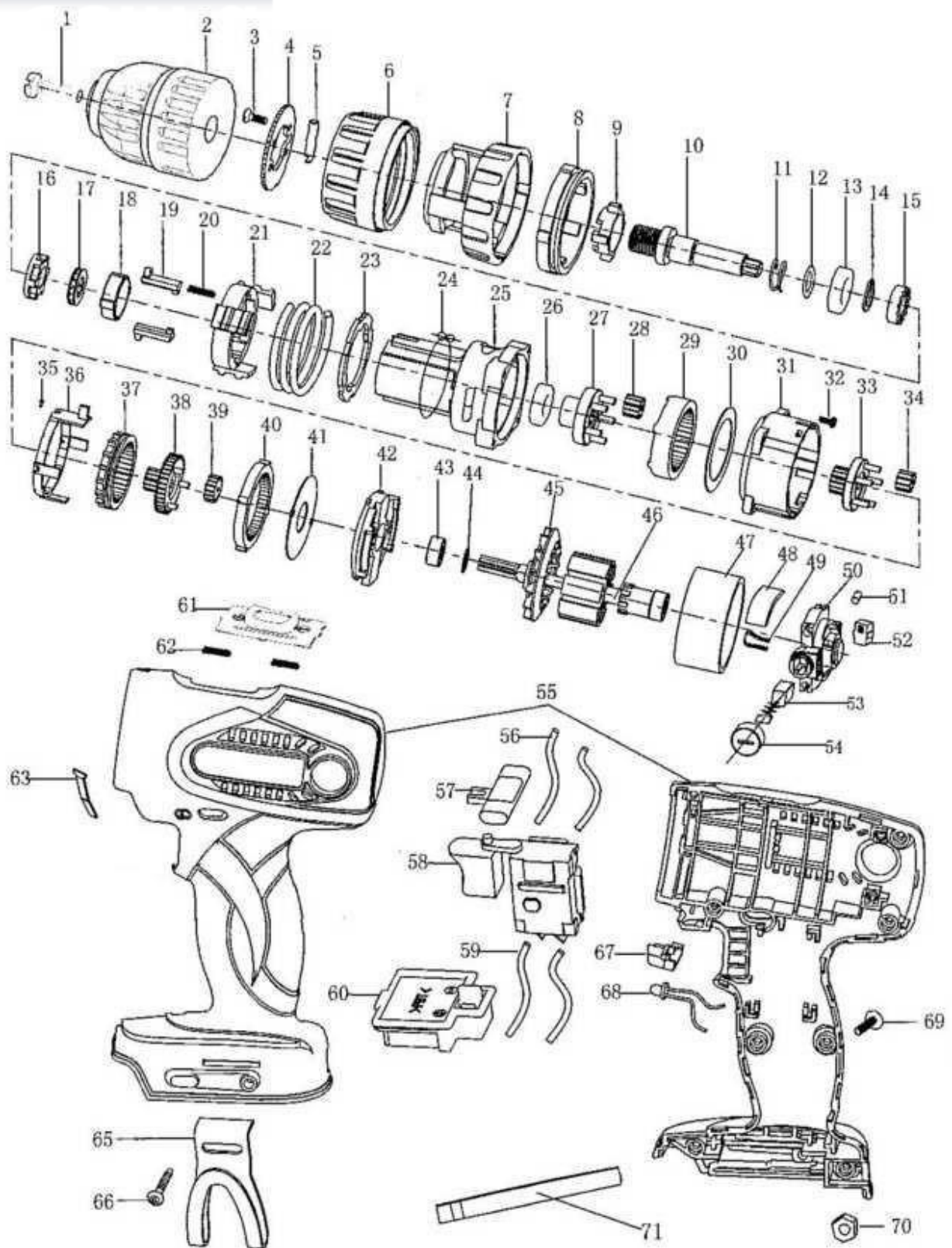
Wiertarko-wkrętarka WAK-Li 18DD
