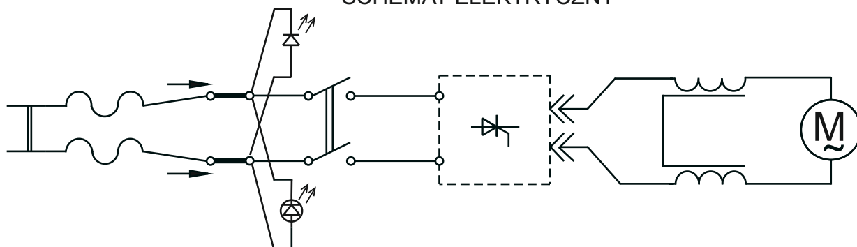
SCHEMAT ELEKTRYCZNY
